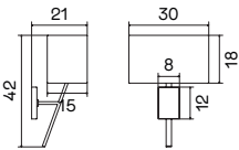
Ref. 151/AP PT Cromado EN Chrome 1 x E27 (B) L8*W12 cm (A) 547 L30*W15*H18 cm L30*W21*H42 cm
