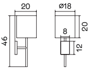
Ref. 003/AP PT Cromado EN Chrome 1 x E27 (B) L12*W8 cm (A) 040 Ø18*H20 cm L20*W18*H46 cm
